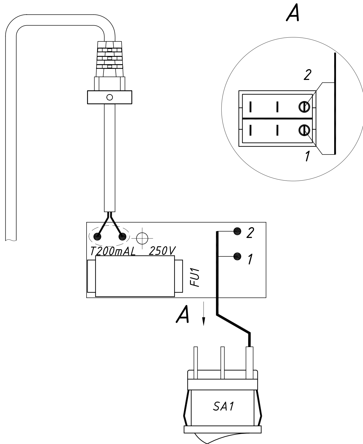
Плата предохранителя Сборочный чертеж
