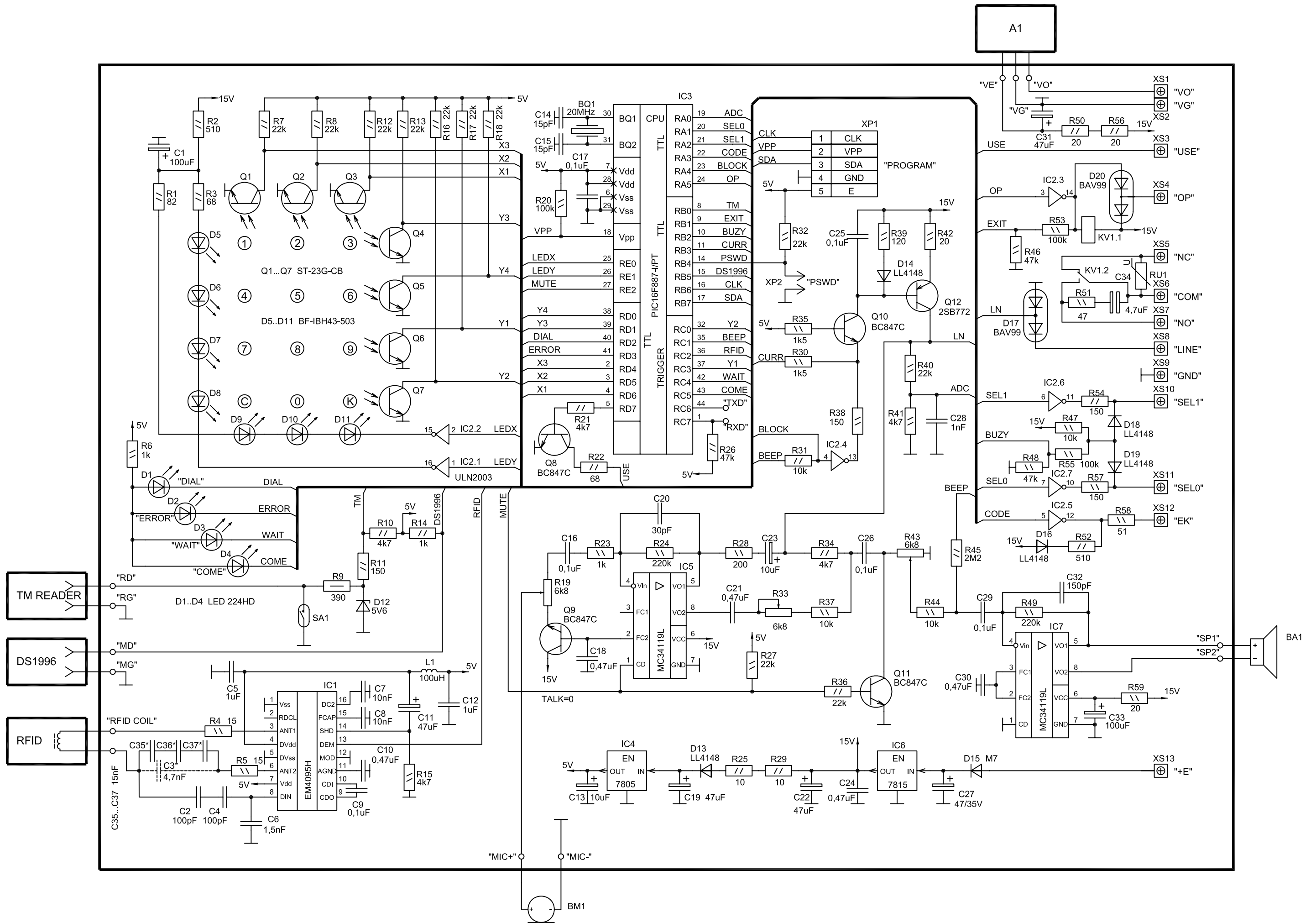
БВД-М200VP Схема электрическая принципиальная
