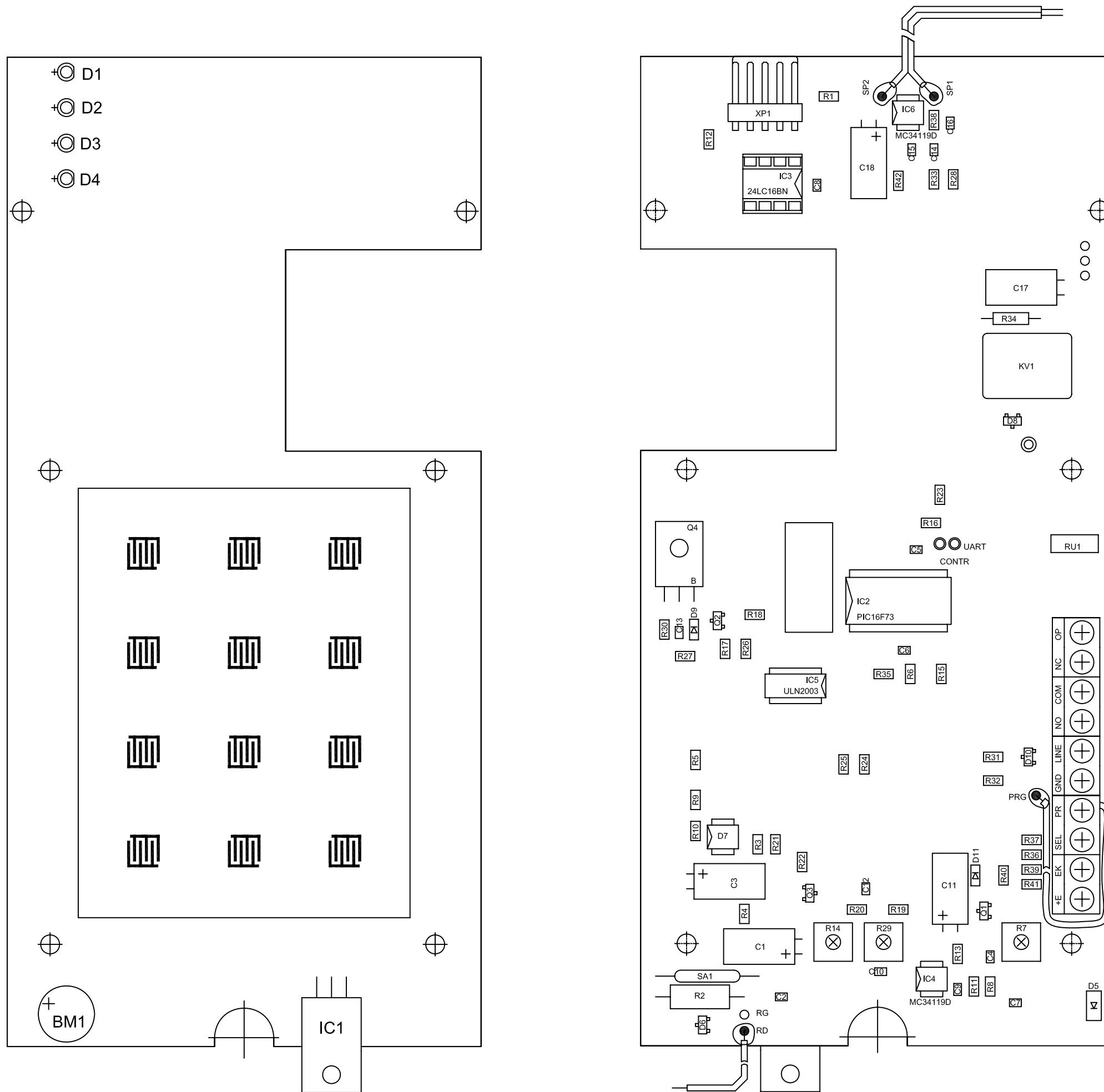
Плата БВД-N100 Сборочный чертеж
