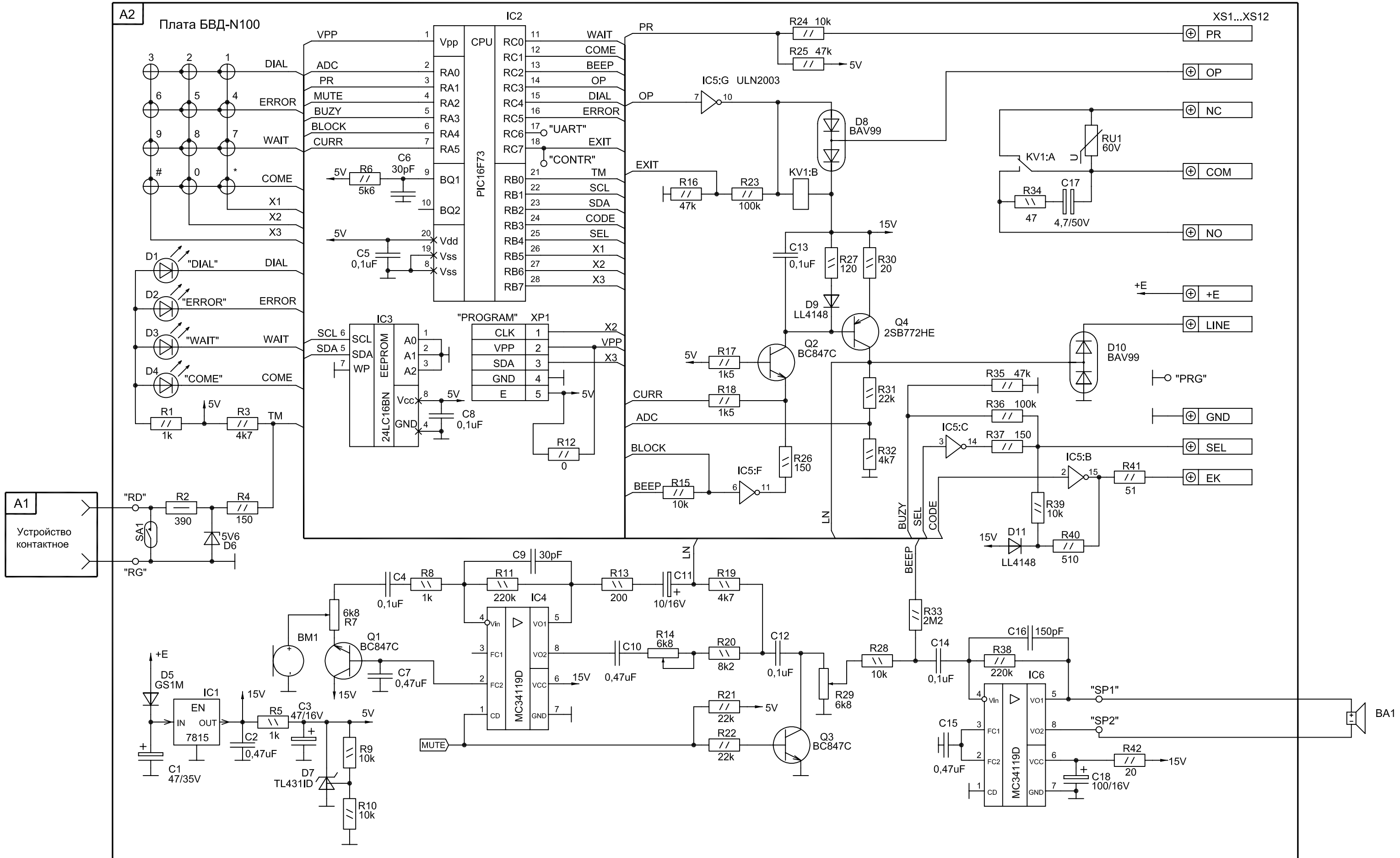
БВД-N100 Схема электрическая принципиальная
