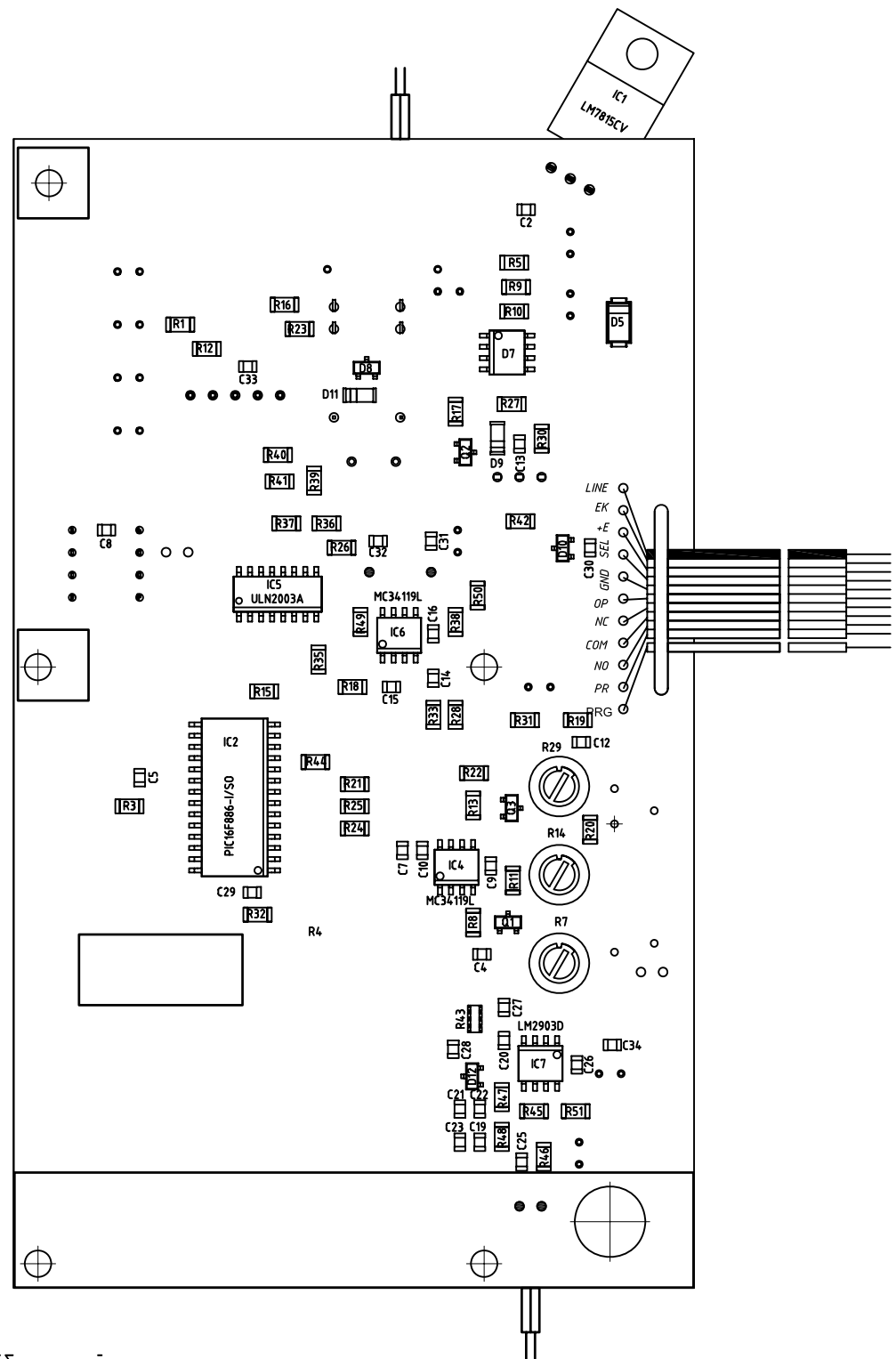
Плата БВД-SM100R Сборный чертёж
