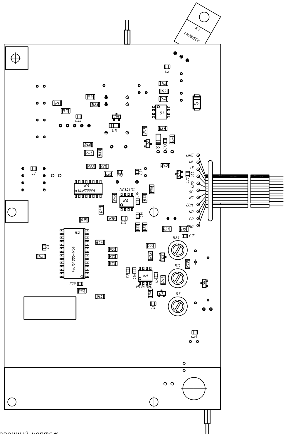
Плата БВД-SM100 Сборочный чертеж
